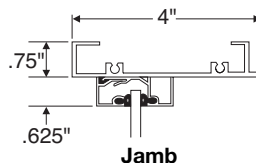
Jamb
